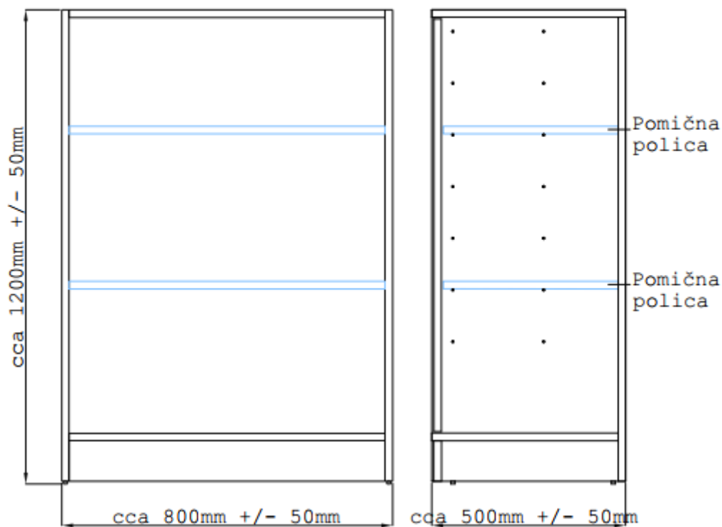
Stavka 5. shema: oprema/namještaj – ormar za odgajatelja
